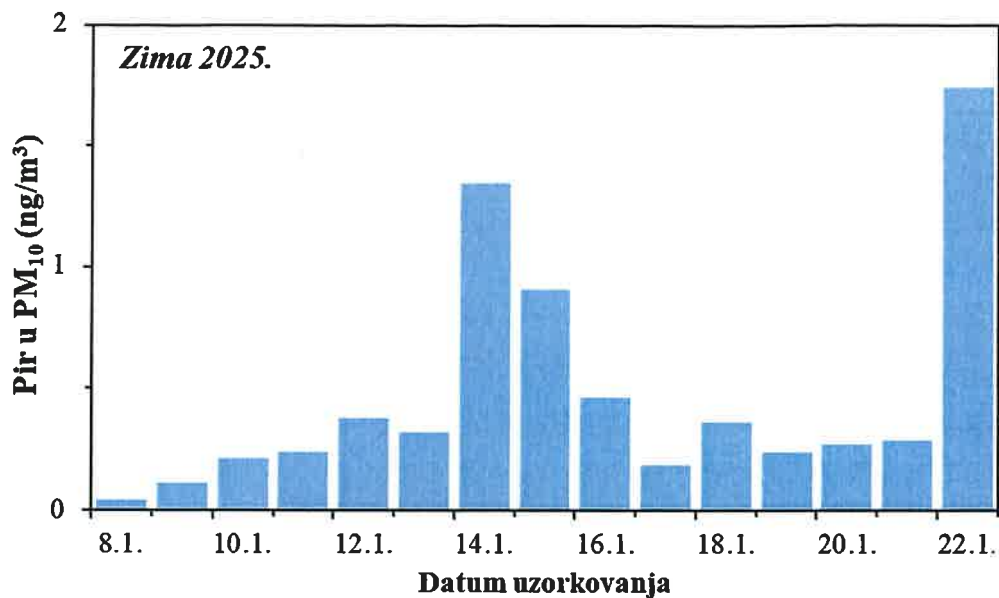
Slika 27. Kretanje srednjih dnevnih koncentracija Pir u PM 10 frakciji lebdećih čestica na imisijskoj mjernoj postaji Jakuševac tijekom zimskog razdoblja 2025. godine
