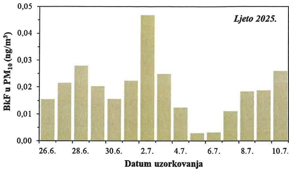
Slika 37. Kretanje srednjih dnevnih koncentracija BkF u PM 10 frakciji lebdećih čestica na imisijskoj mjernejoj postaji Jakuševac tijekom ljetnog razdoblja 2025. godine
