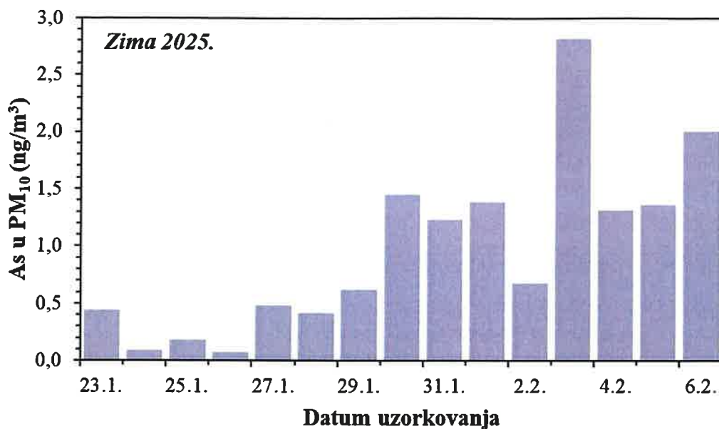
Slika 15. Kretanje srednjih dnevnih koncentracija arsena u PM 10 frakciji lebdećih čestica na imisijskoj mjernoj postaji Jakuševac tijekom zimskog razdoblja 2025. godine
