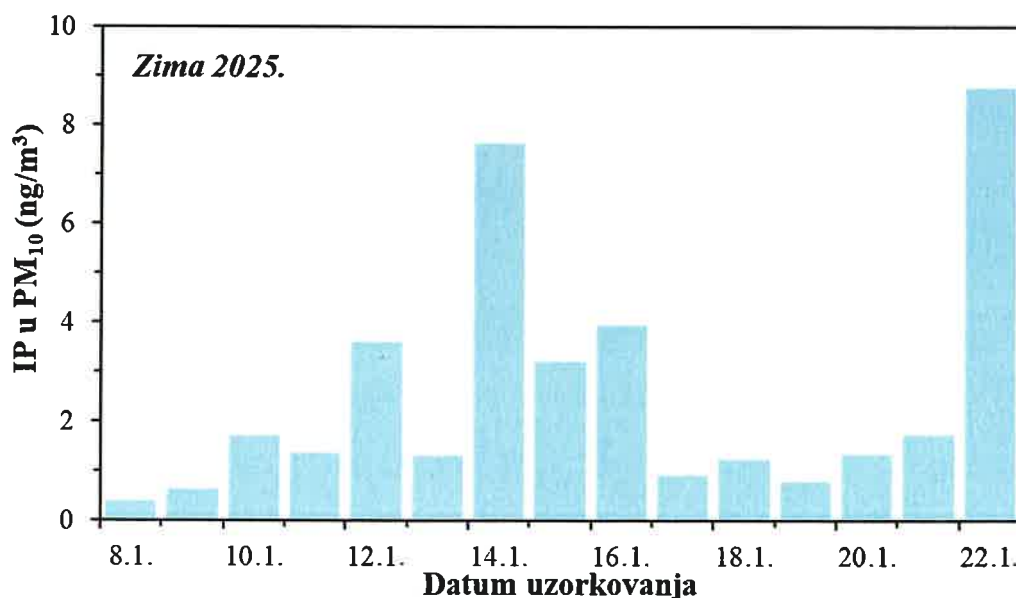
Slika 47. Kretanje srednjih dnevnih koncentracija IP u PM 10 frakciji lebdećih čestica na imisijskoj mjernoj postaji Jakuševac tijekom zimskog razdoblja 2025. godine
