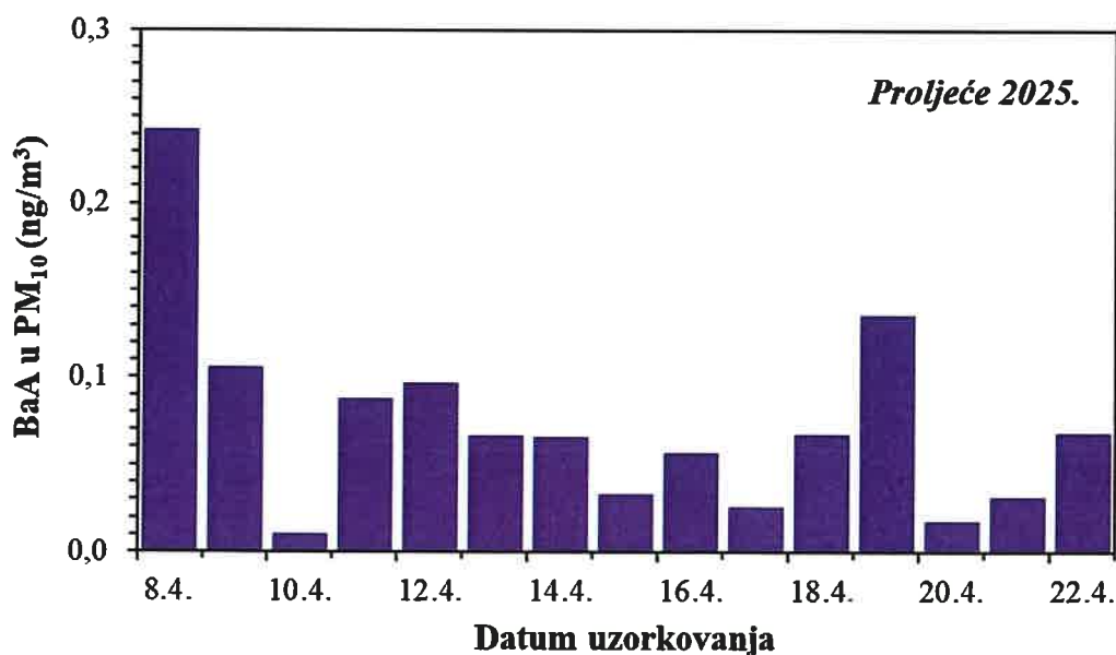
Slika 52. Kretanje srednjih dnevnih koncentracija BaAnt u PM 10 frakciji lebdećih čestica na imisijskoj mjernoj postaji Jakuševac tijekom proljetnog razdoblja 2025. godine
