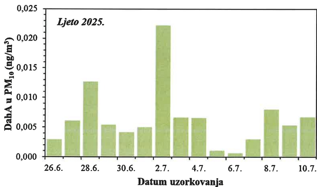
Slika 41. Kretanje srednjih dnevnih koncentracija DahA u PM 10 frakciji lebdećih čestica na imisijskoj mjernejoj postaji Jakuševac tijekom ljetnog razdoblja 2025. godine
