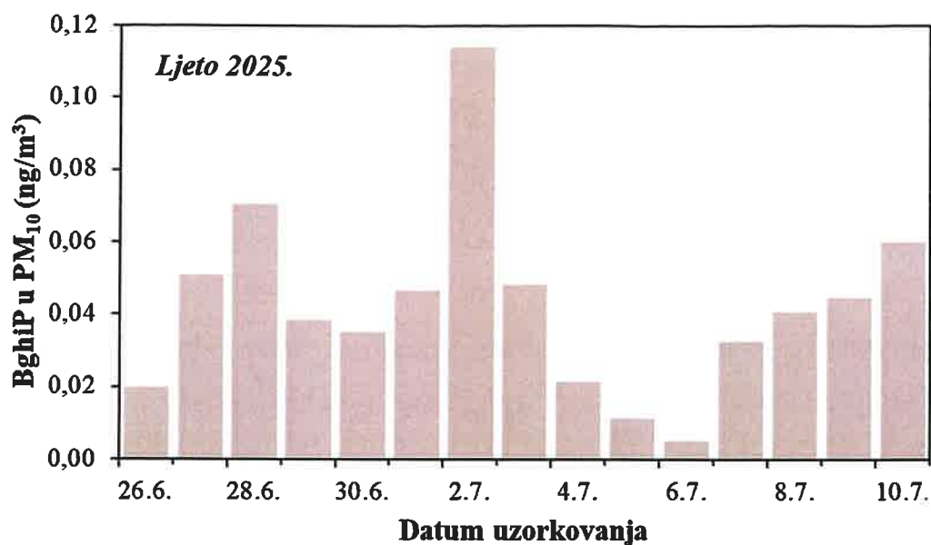
Slika 45. Kretanje srednjih dnevnih koncentracija BghiP u PM 10 frakciji lebdećih čestica na imisijskoj mjernoj postaji Jakuševac tijekom ljetnog razdoblja 2025. godine
