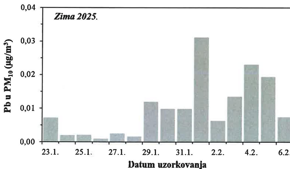
Slika 3. Kretanje srednjih dnevnih koncentracija olova u PM 10 frakciji lebdećih čestica na imisijskoj mjernejoj postaji Jakuševac tijekom zimskog razdoblja 2025. godine
