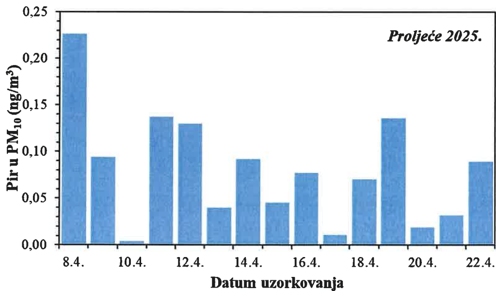
Slika 28. Kretanje srednjih dnevnih koncentracija Pir u PM 10 frakciji lebdećih čestica na imisijskoj mjernoj postaji Jakuševac tijekom proljetnog razdoblja 2025. godine
