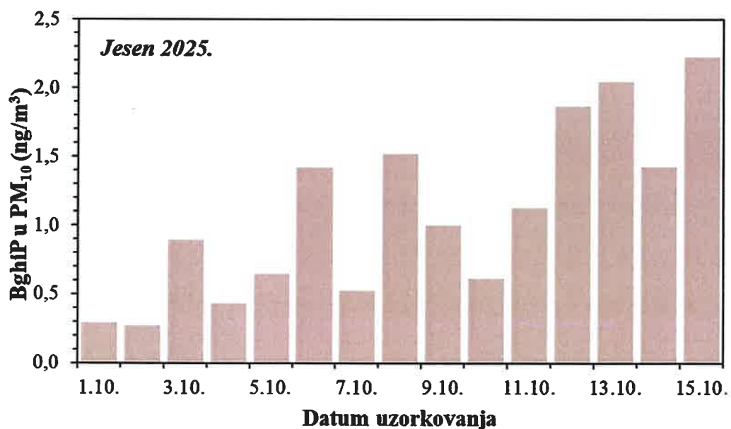
Slika 46. Kretanje srednjih dnevnih koncentracija BghiP u PM 10 frakciji lebdećih čestica na imisijskoj mjernoj postaji Jakuševac tijekom jesenskog razdoblja 2025. godine
