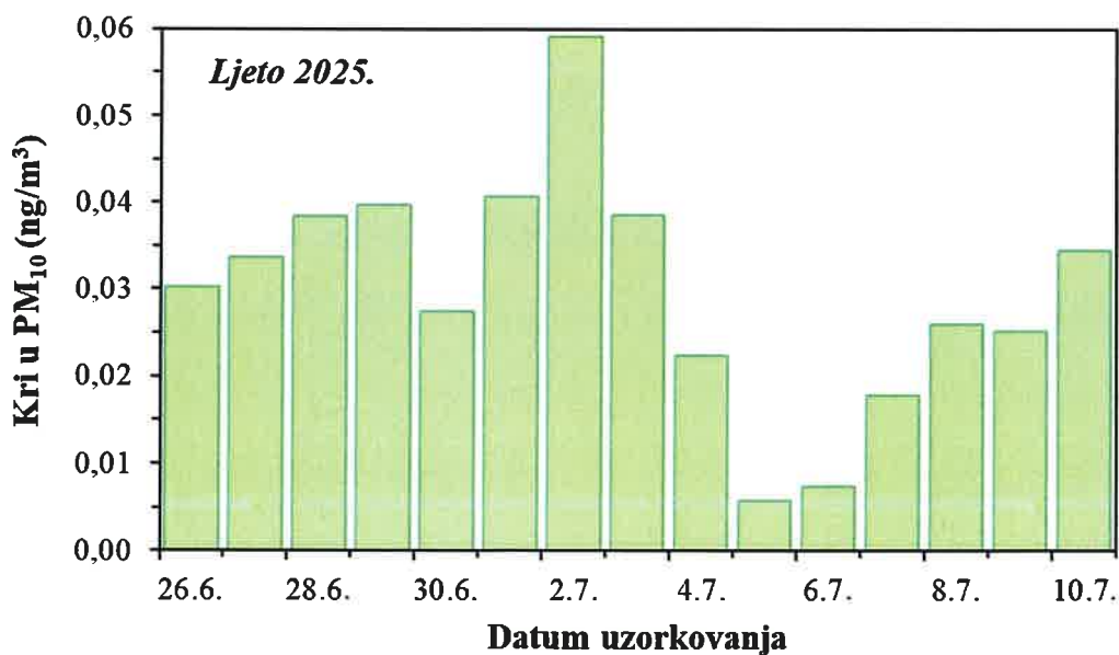
Slika 57. Kretanje srednjih dnevnih koncentracija Kri u PM 10 frakciji lebdećih čestica na imisijskoj mjernejoj postaji Jakuševac tijekom ljetnog razdoblja 2025. godine
