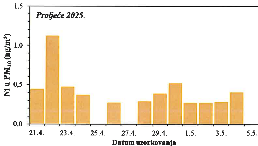
Slika 8. Kretanje srednjih dnevnih koncentracija nikla u PM 10 frakciji lebdećih čestica na imisijskoj mjernoj postaji Jakuševac tijekom proljetnog razdoblja 2025. godine
