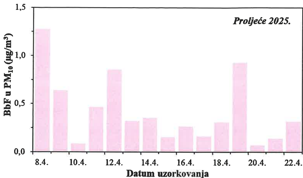
Slika 32. Kretanje srednjih dnevnih koncentracija BbF u PM 10 frakciji lebdećih čestica na imisijskoj mjernoj postaji Jakuševac tijekom proljetnog razdoblja 2025. godine
