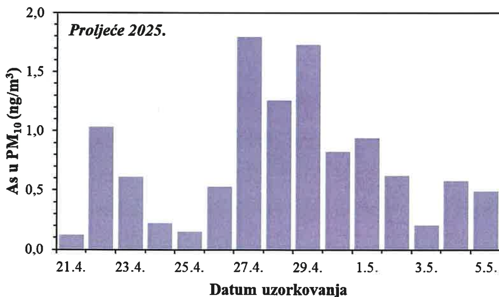
Slika 16. Kretanje srednjih dnevnih koncentracija arsena u PM 10 frakciji lebdećih čestica na imisijskoj mjernoj postaji Jakuševac tijekom proljetnog razdoblja 2025. godine
