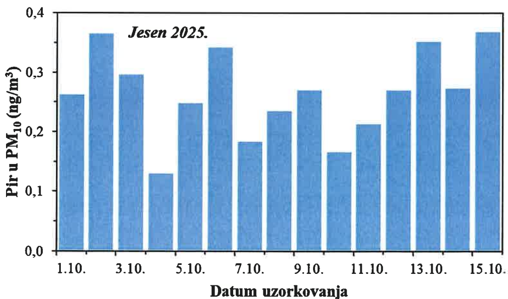
Slika 30. Kretanje srednjih dnevnih koncentracija Pir u PM 10 frakciji lebdećih čestica na imisijskoj mjernoj postaji Jakuševac tijekom jesenskog razdoblja 2025. godine
