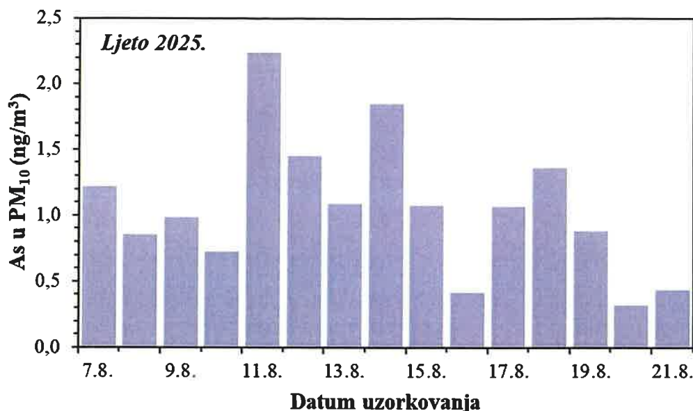
Slika 17. Kretanje srednjih dnevnih koncentracija arsena u PM 10 frakciji lebdećih čestica na imisijskoj mjernejoj postaji Jakuševac tijekom ljetnog razdoblja 2025. godine
