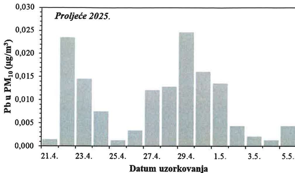
Slika 4. Kretanje srednjih dnevnih koncentracija olova u PM 10 frakciji lebdećih čestica na imisijskoj mjernoj postaji Jakuševac tijekom proljetnog razdoblja 2025. godine
