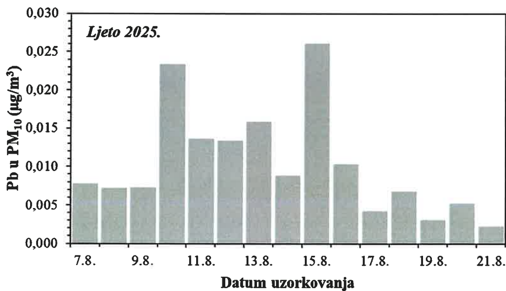
Slika 5. Kretanje srednjih dnevnih koncentracija olova u PM 10 frakciji lebdećih čestica na imisijskoj mjernoj postaji Jakuševac tijekom ljetnog razdoblja 2025. godine
