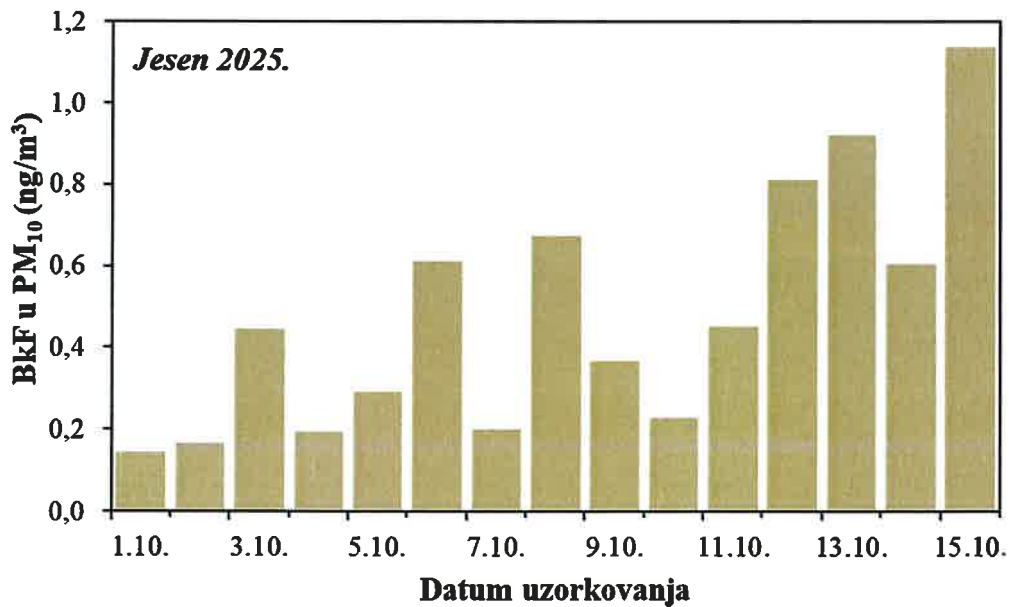
Slika 38. Kretanje srednjih dnevnih koncentracija BkF u PM 10 frakciji lebdećih čestica na imisijskoj mjernejoj postaji Jakuševac tijekom jesenskog razdoblja 2025. godine
