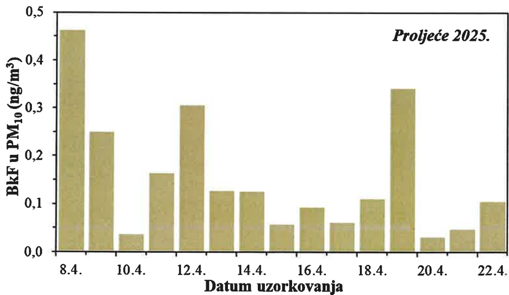
Slika 36. Kretanje srednjih dnevnih koncentracija BkF u PM 10 frakciji lebdećih čestica na imisijskoj mjernejoj postaji Jakuševac tijekom proljetnog razdoblja 2025. godine
