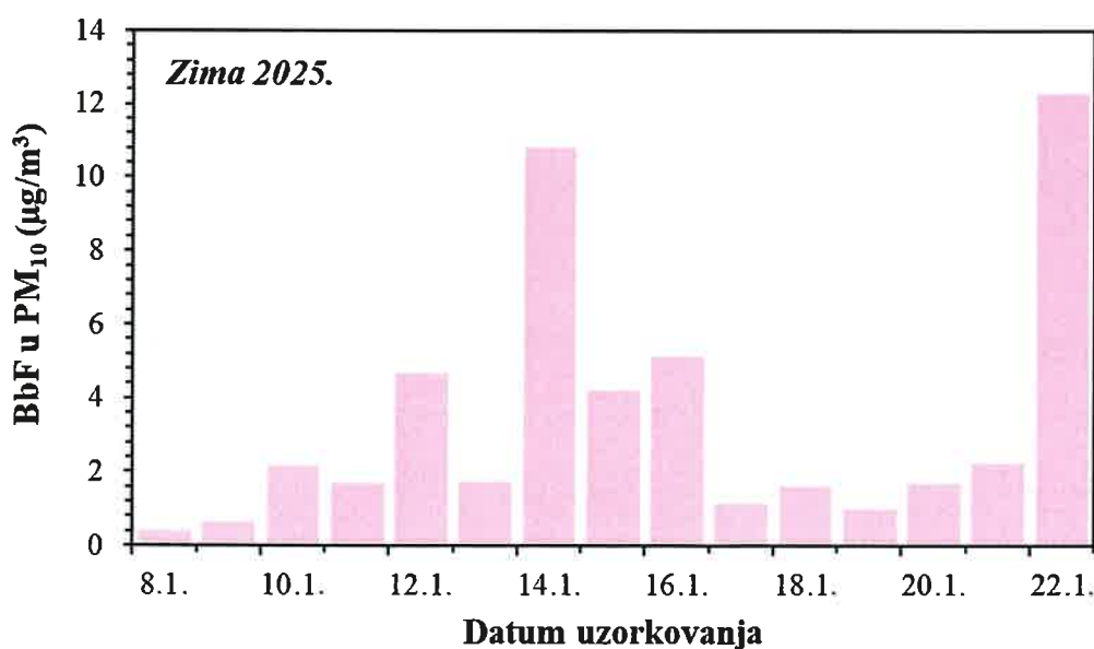
Slika 31. Kretanje srednjih dnevnih koncentracija BbF u PM 10 frakciji lebdećih čestica na imisijskoj mjernoj postaji Jakuševac tijekom zimskog razdoblja 2025. godine
