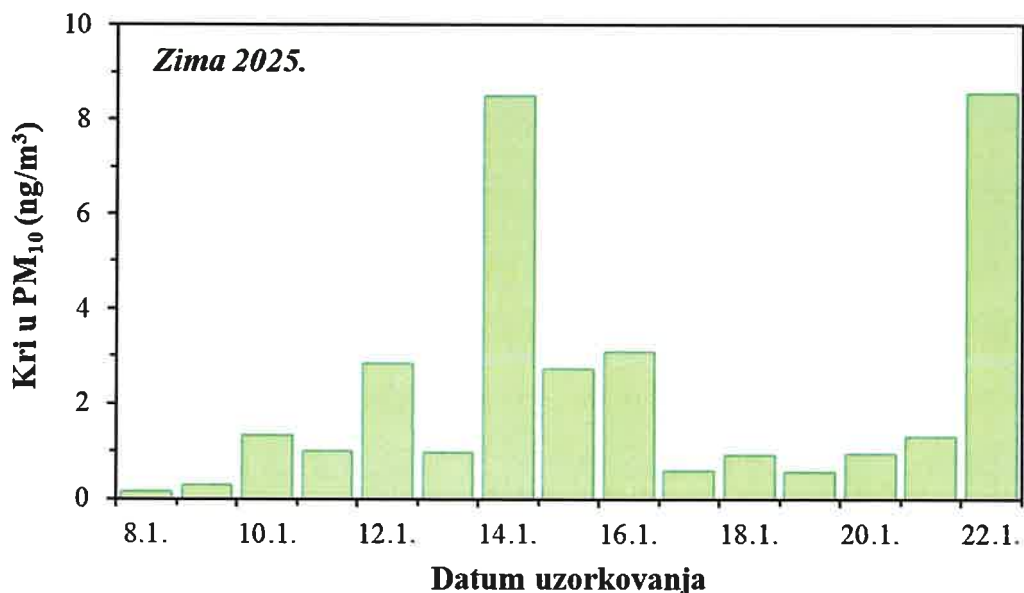
Slika 55. Kretanje srednjih dnevnih koncentracija Kri u PM 10 frakciji lebdećih čestica na imisijskoj mjernoj postaji Jakuševac tijekom zimskog razdoblja 2025. godine
