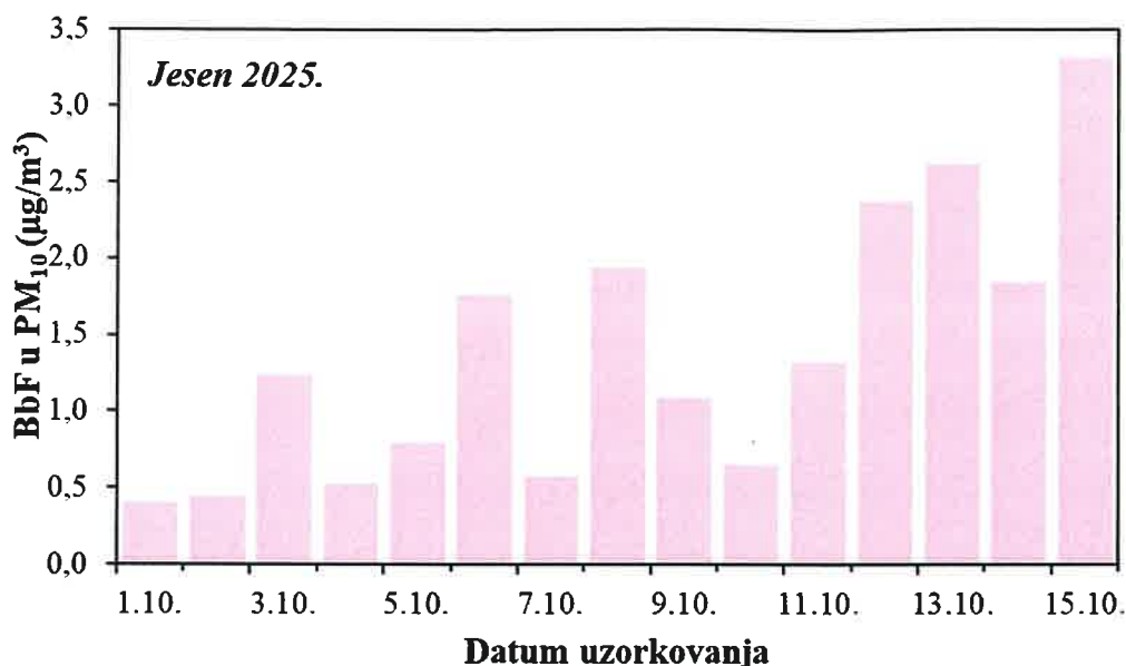
Slika 34. Kretanje srednjih dnevnih koncentracija BbF u PM 10 frakciji lebdećih čestica na imisijskoj mjernoj postaji Jakuševac tijekom jesenskog razdoblja 2025. godine
