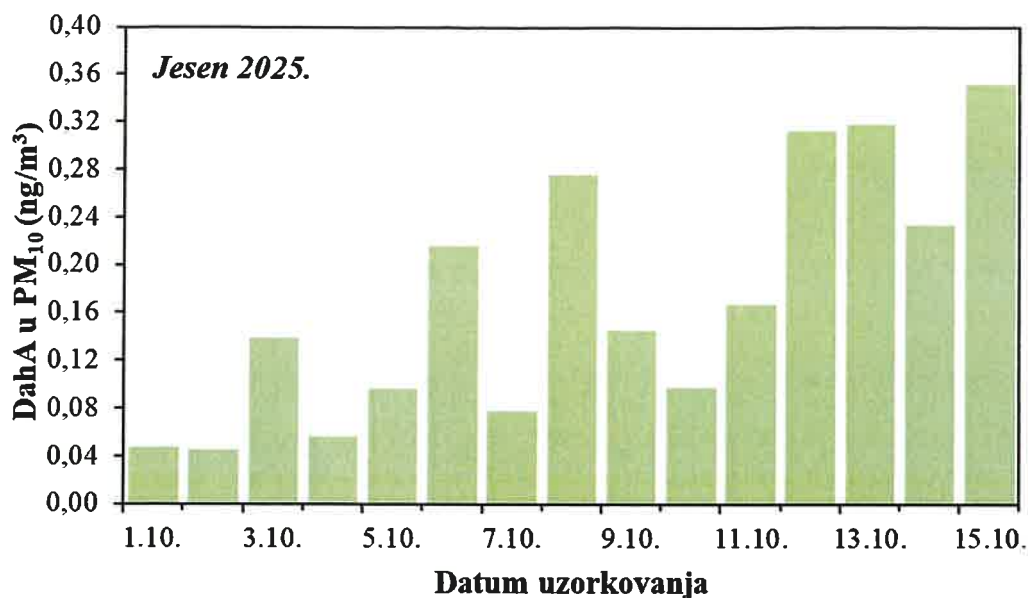
Slika 42. Kretanje srednjih dnevnih koncentracija DahA u PM 10 frakciji lebdećih čestica na imisijskoj mornoj postaji Jakuševac tijekom jesenskog razdoblja 2025. godine
