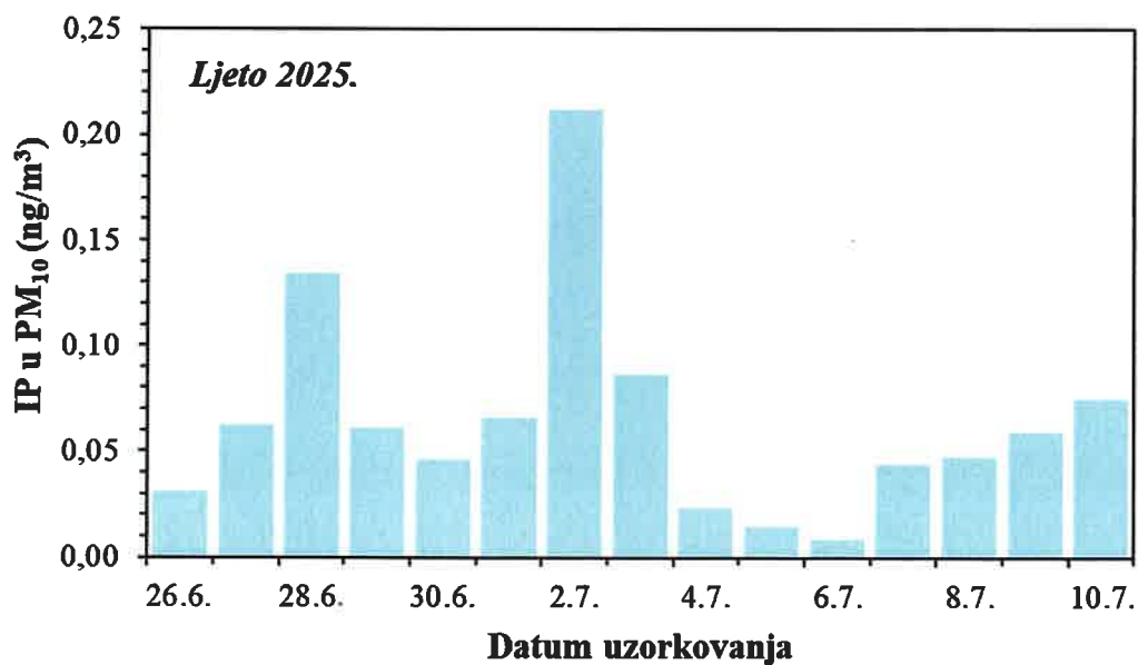
Slika 49. Kretanje srednjih dnevnih koncentracija IP u PM 10 frakciji lebdećih čestica na imisijskoj mjernoj postaji Jakuševac tijekom ljetnog razdoblja 2025. godine
