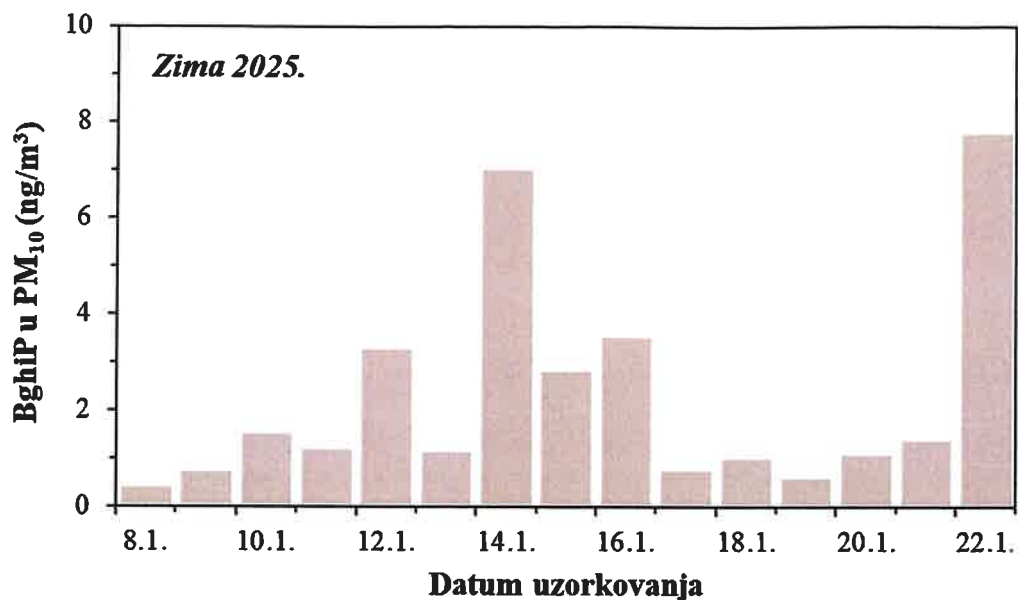
Slika 43. Kretanje srednjih dnevnih koncentracija BghiP u PM 10 frakciji lebdećih čestica na imisijskoj mjernejoj postaji Jakuševac tijekom zimskog razdoblja 2025. godine
