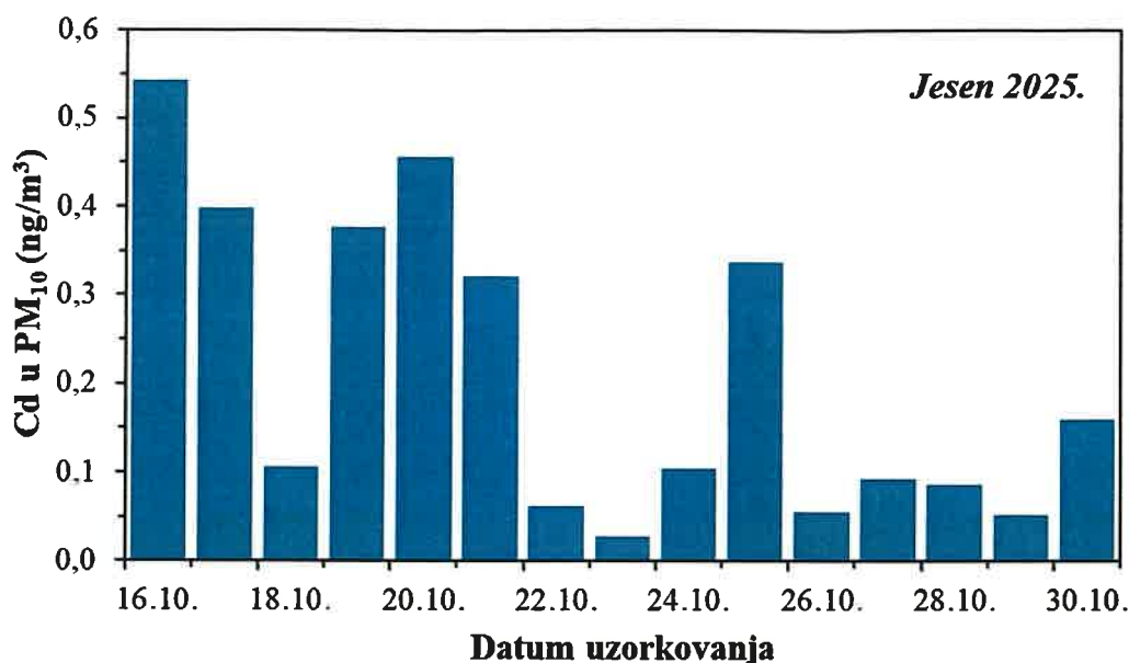
Slika 14. Kretanje srednjih dnevnih koncentracija kadmija u PM 10 frakciji lebdećih čestica na imisijskoj mjernoj postaji Jakusevec tijekom jesenskog razdoblja 2025. godine
