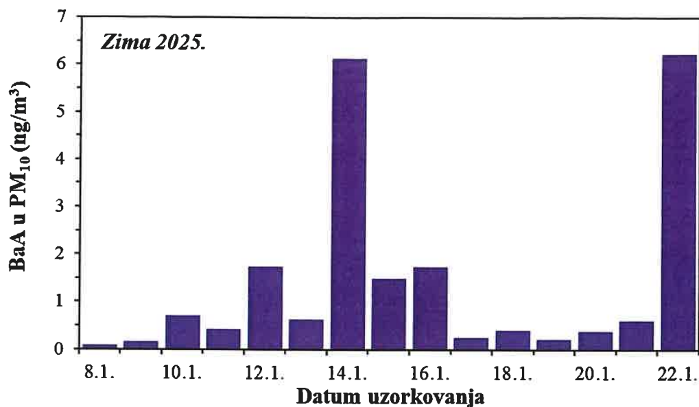
Slika 51. Kretanje srednjih dnevnih koncentracija BaA u PM 10 frakciji lebdećih čestica na imisijskoj mjernoj postaji Jakuševac tijekom zimskog razdoblja 2025. godine
