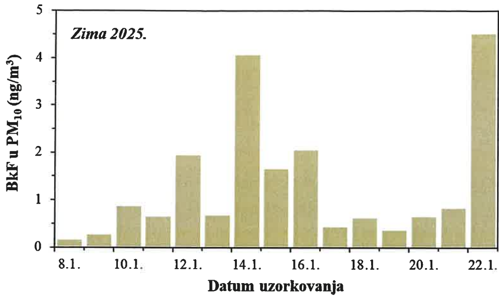
Slika 35. Kretanje srednjih dnevnih koncentracija BkF u PM 10 frakciji lebdećih čestica na imisijskoj mjernejoj postaji Jakuševac tijekom zimskog razdoblja 2025. godine
