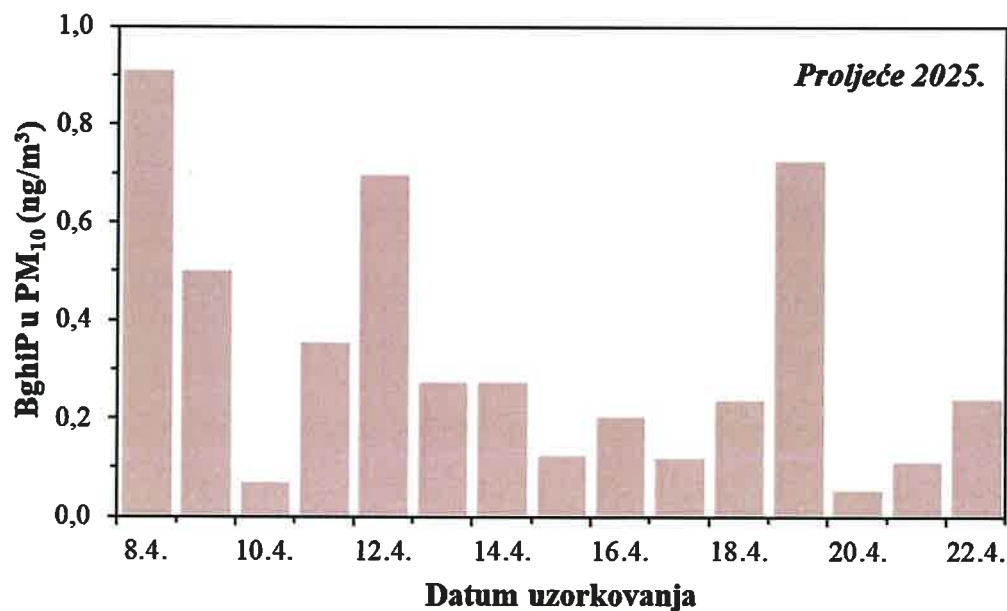
Slika 44. Kretanje srednjih dnevnih koncentracija BghiP u PM 10 frakciji lebdećih čestica na imisijskoj mjernejoj postaji Jakuševac tijekom proljetnog razdoblja 2025. godine
