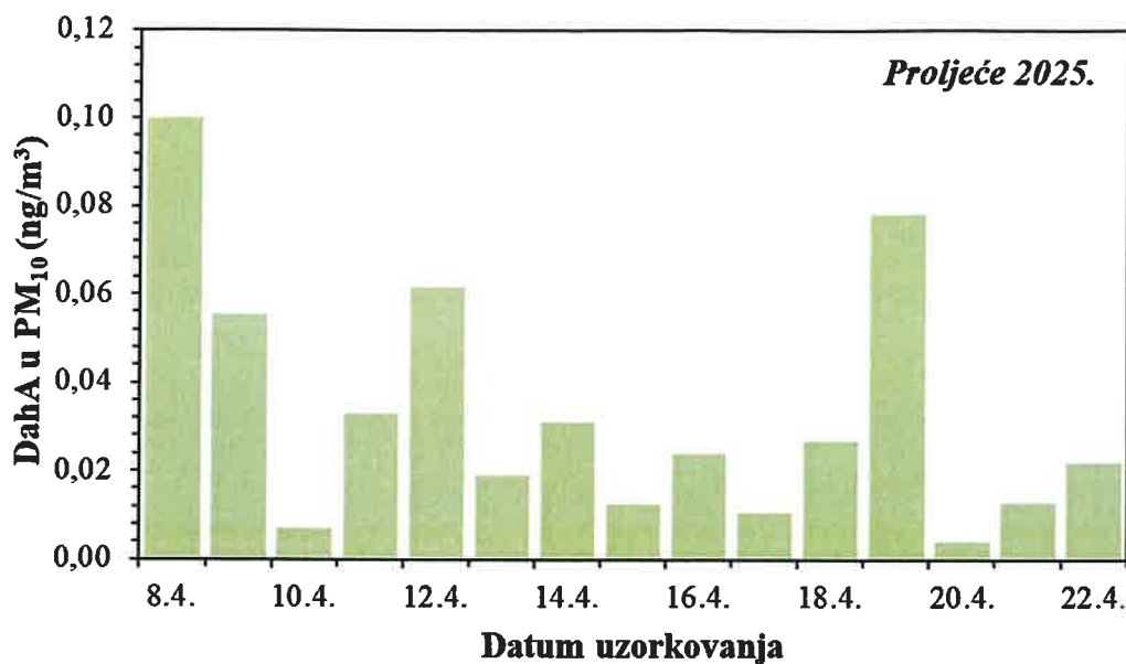
Slika 40. Kretanje srednjih dnevnih koncentracija DahA u PM 10 frakciji lebdećih čestica na imisijskoj mjernejoj postaji Jakuševac tijekom proljetnog razdoblja 2025. godine
