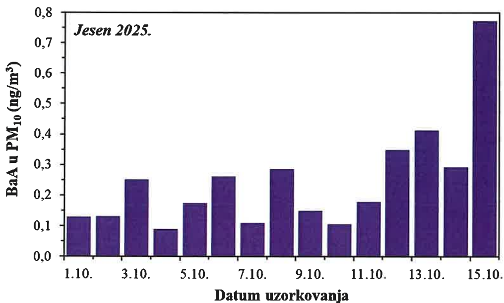
Slika 54. Kretanje srednjih dnevnih koncentracija BaAnt u PM 10 frakciji lebdećih čestica na imisijskoj mjernoj postaji Jakuševac tijekom jesenskog razdoblja 2025. godine
