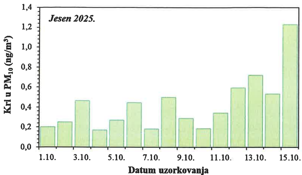
Slika 58. Kretanje srednjih dnevnih koncentracija Kri u PM 10 frakciji lebdećih čestica na imisijskoj mjernoj postaji Jakuševac tijekom jesenskog razdoblja 2025. godine
