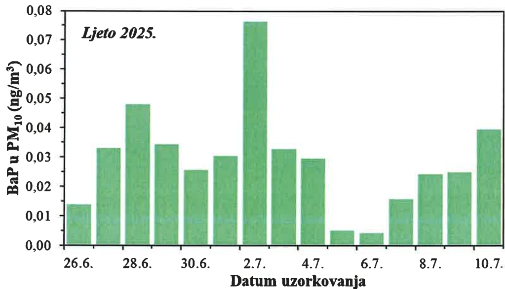
Slika 21. Kretanje srednjih dnevnih koncentracija BaP u PM 10 frakciji lebdećih čestica na imisijskoj mjernoj postaji Jakuševac tijekom ljetnog razdoblja 2025. godine
