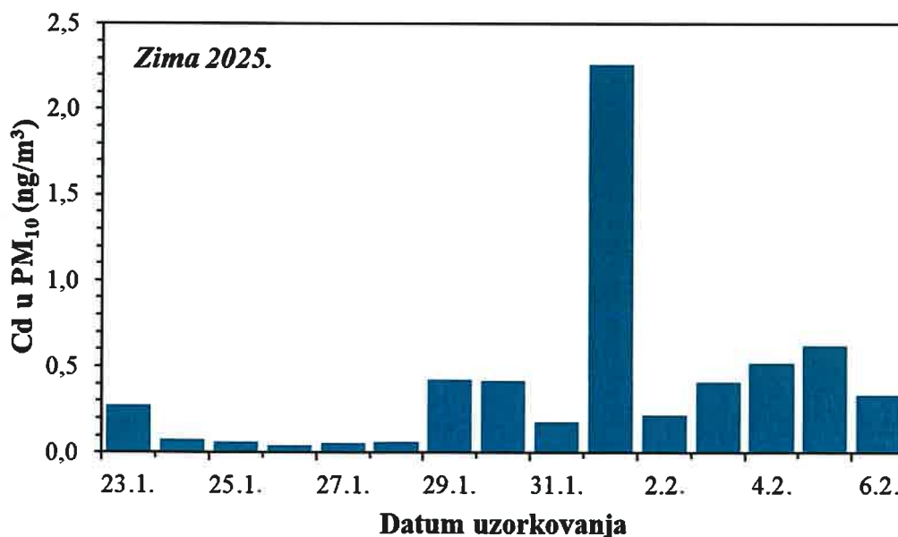
Slika 11. Kretanje srednjih dnevnih koncentracija kadmija u PM 10 frakciji lebdećih čestica na imisijskoj mjernoj postaji Jakuševac tijekom zimskog razdoblja 2025. godine
