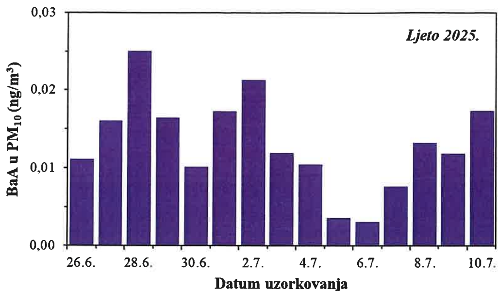
Slika 53. Kretanje srednjih dnevnih koncentracija BaAnt u PM 10 frakciji lebdećih čestica na imisijskoj mjernoj postaji Jakuševac tijekom ljetnog razdoblja 2025. godine
