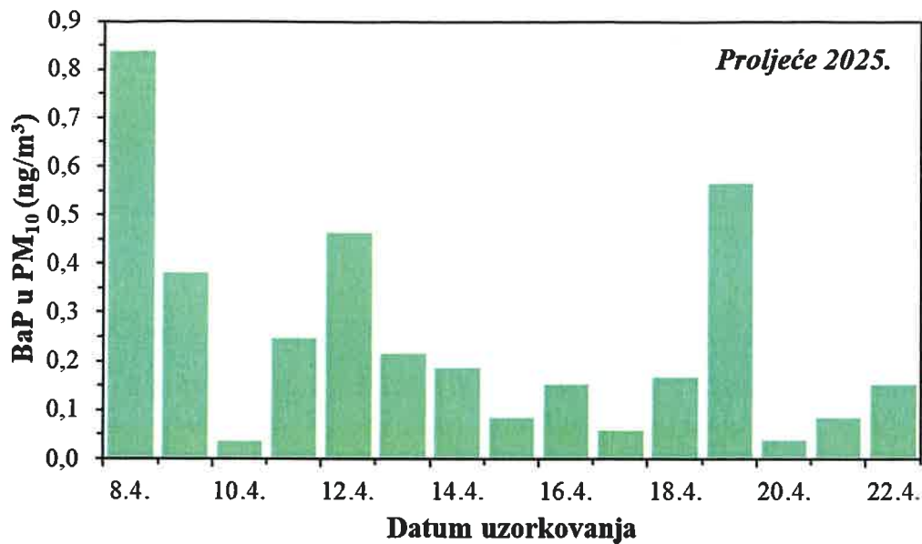
Slika 20. Kretanje srednjih dnevnih koncentracija BaP u PM 10 frakciji lebdećih čestica na imisijskoj mjernoj postaji Jakuševac tijekom proljetnog razdoblja 2025. godine
