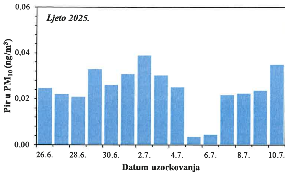
Slika 29. Kretanje srednjih dnevnih koncentracija Pir u PM 10 frakciji lebdećih čestica na imisijskoj mjernoj postaji Jakuševac tijekom ljetnog razdoblja 2025. godine
