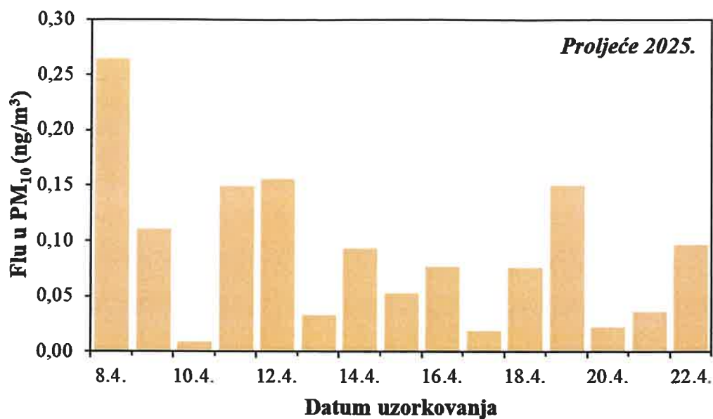
Slika 24. Kretanje srednjih dnevnih koncentracija Flu u PM 10 frakciji lebdećih čestica na imisijskoj mjernejoj postaji Jakuševac tijekom proljetnog razdoblja 2025. godine
