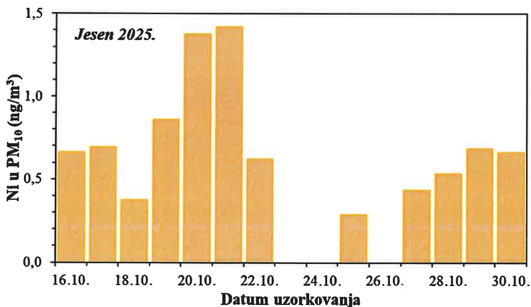
Slika 10. Kretanje srednjih dnevnih koncentracija nikla u PM 10 frakciji lebdećih čestica na imisijskoj mjernoj postaji Jakuševac tijekom jesenskog razdoblja 2025. godine
