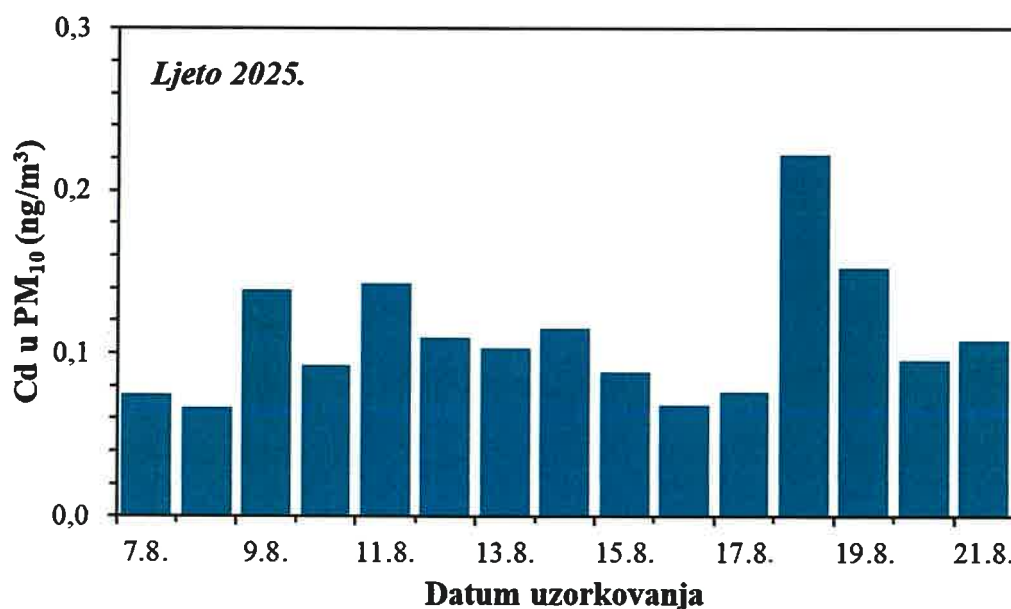
Slika 13. Kretanje srednjih dnevnih koncentracija kadmija u PM 10 frakciji lebdećih čestica na imisijskoj mjernoj postaji Jakuševac tijekom ljetnog razdoblja 2025. godine
