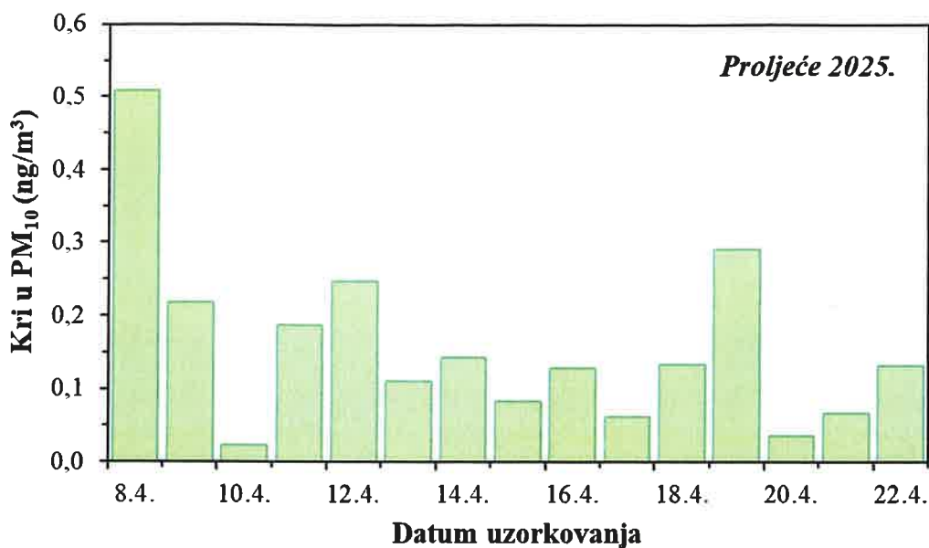
Slika 56. Kretanje srednjih dnevnih koncentracija Kri u PM 10 frakciji lebdećih čestica na imisijskoj mjernejoj postaji Jakuševac tijekom proljetnog razdoblja 2025. godine
