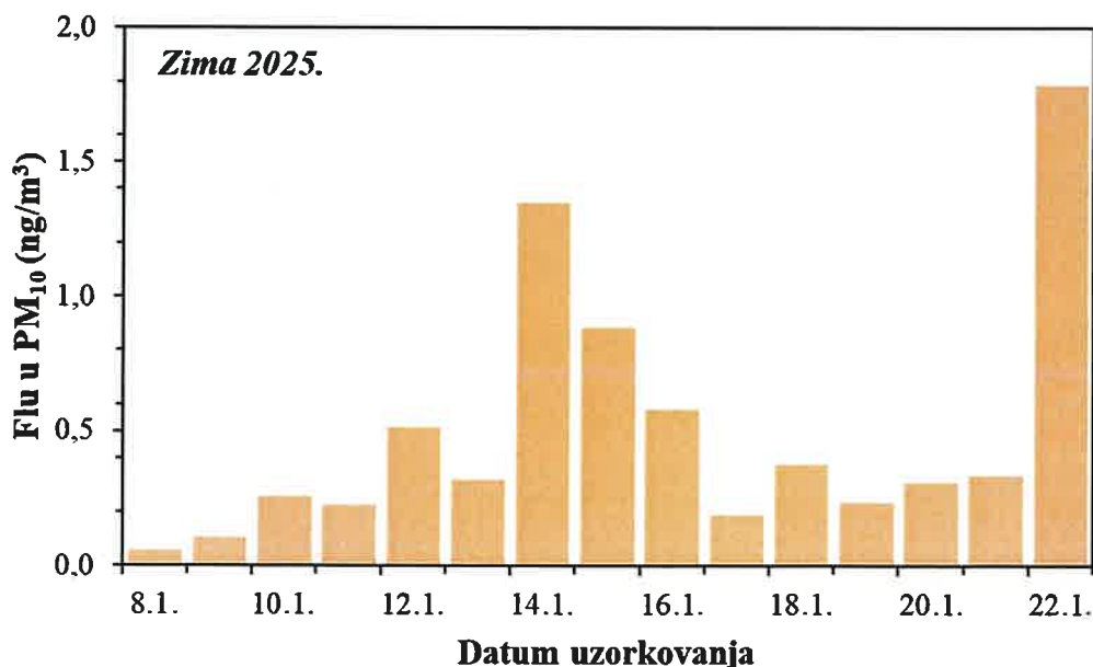
Slika 23. Kretanje srednjih dnevnih koncentracija Flu u PM 10 frakciji lebdećih čestica na imisijskoj mjernejoj postaji Jakuševac tijekom zimskog razdoblja 2025. godine
