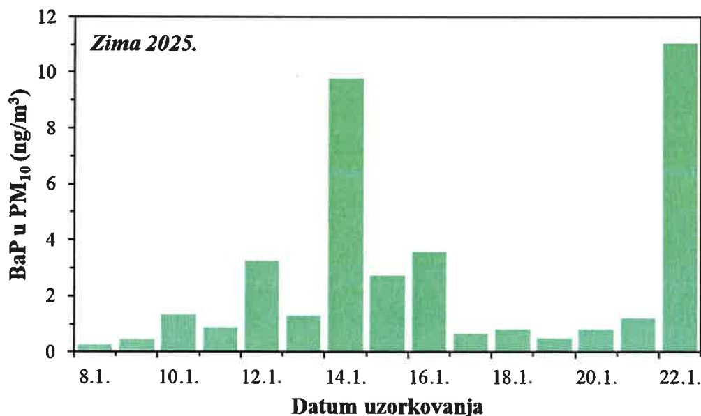
Slika 19. Kretanje srednjih dnevnih koncentracija BaP u PM 10 frakciji lebdećih čestica na imisijskoj mjernoj postaji Jakuševac tijekom zimskog razdoblja 2025. godine
