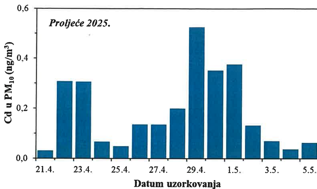
Slika 12. Kretanje srednjih dnevnih koncentracija kadmija u PM 10 frakciji lebdećih čestica na imisijskoj mjernoj postaji Jakuševac tijekom proljetnog razdoblja 2025. godine
