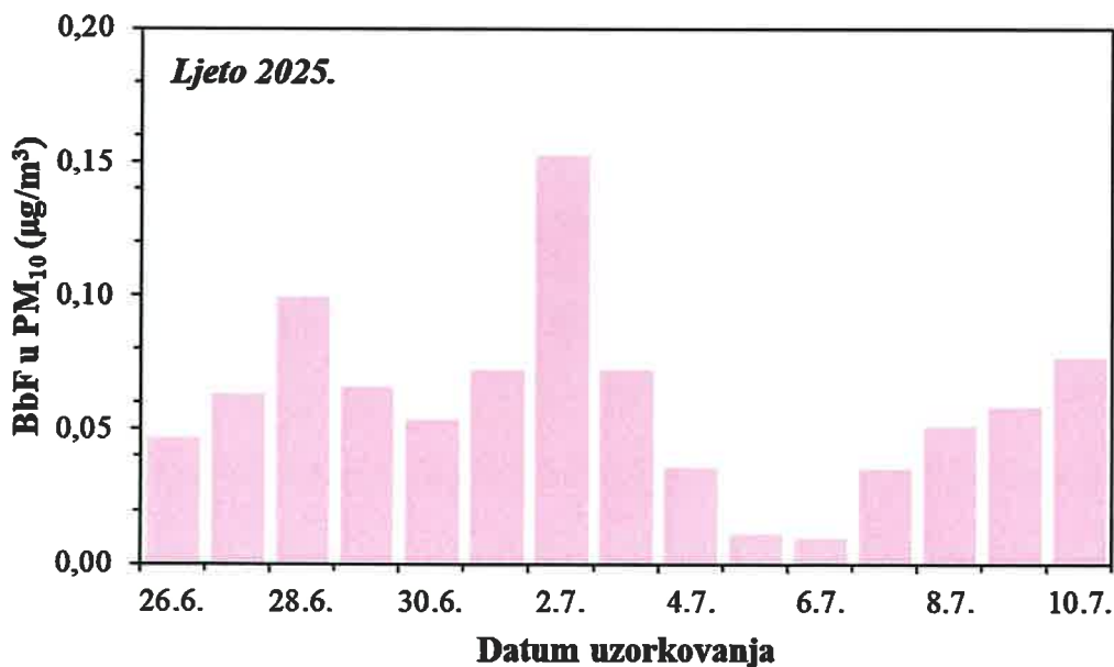
Slika 33. Kretanje srednjih dnevnih koncentracija BbF u PM 10 frakciji lebdećih čestica na imisijskoj mjernoj postaji Jakuševac tijekom ljetnog razdoblja 2025. godine
