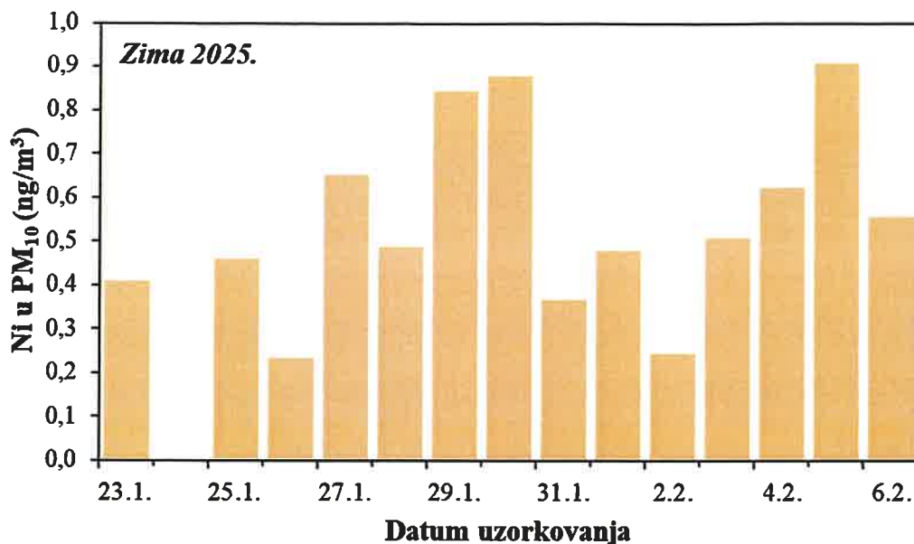
Slika 7. Kretanje srednjih dnevnih koncentracija nikla u PM 10 frakciji lebdećih čestica na imisijskoj mjernoj postaji Jakuševac tijekom zimskog razdoblja 2025. godine
