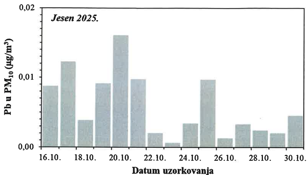
Slika 6. Kretanje srednjih dnevnih koncentracija olova u PM 10 frakciji lebdećih čestica na imisijskoj mjernoj postaji Jakuševac tijekom jesenskog razdoblja 2025. godine
