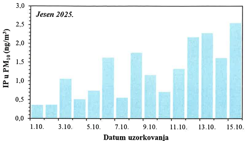
Slika 50. Kretanje srednjih dnevnih koncentracija IP u PM 10 frakciji lebdećih čestica na imisijskoj mjernoj postaji Jakuševac tijekom jesenskog razdoblja 2025. godine
