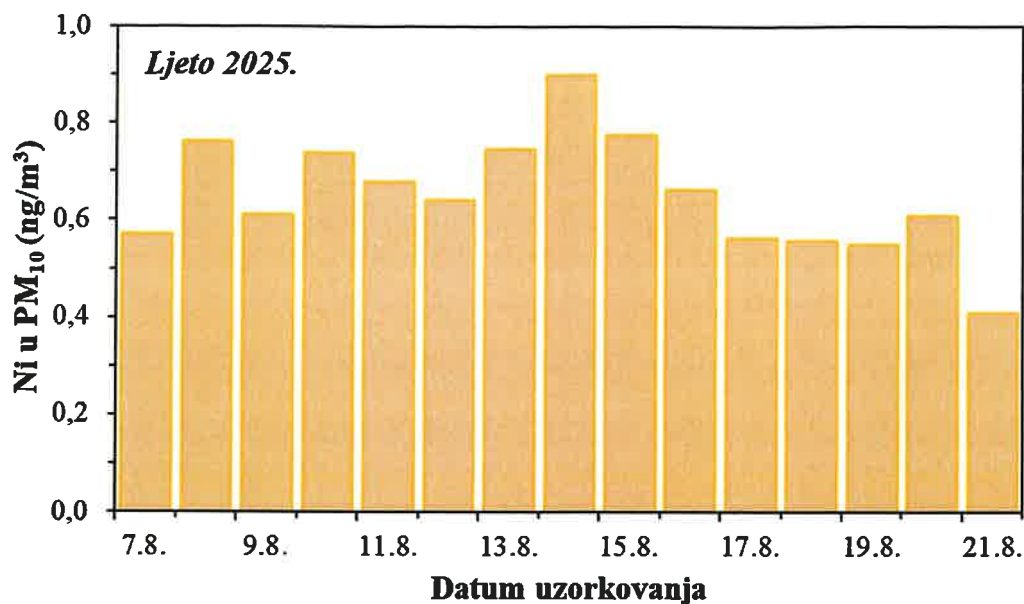
Slika 9. Kretanje srednjih dnevnih koncentracija nikla u PM 10 frakciji lebdećih čestica na imisijskoj mjernoj postaji Jakuševac tijekom ljetnog razdoblja 2025. godine
