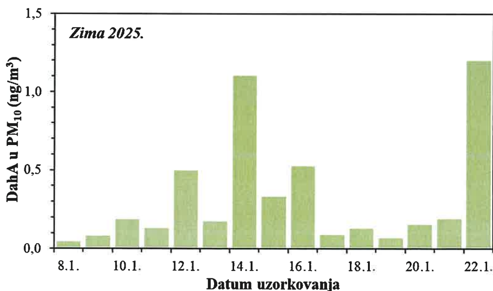
Slika 39. Kretanje srednjih dnevnih koncentracija DahA u PM 10 frakciji lebdećih čestica na imisijskoj mjernoj postaji Jakuševac tijekom zimskog razdoblja 2025. godine
