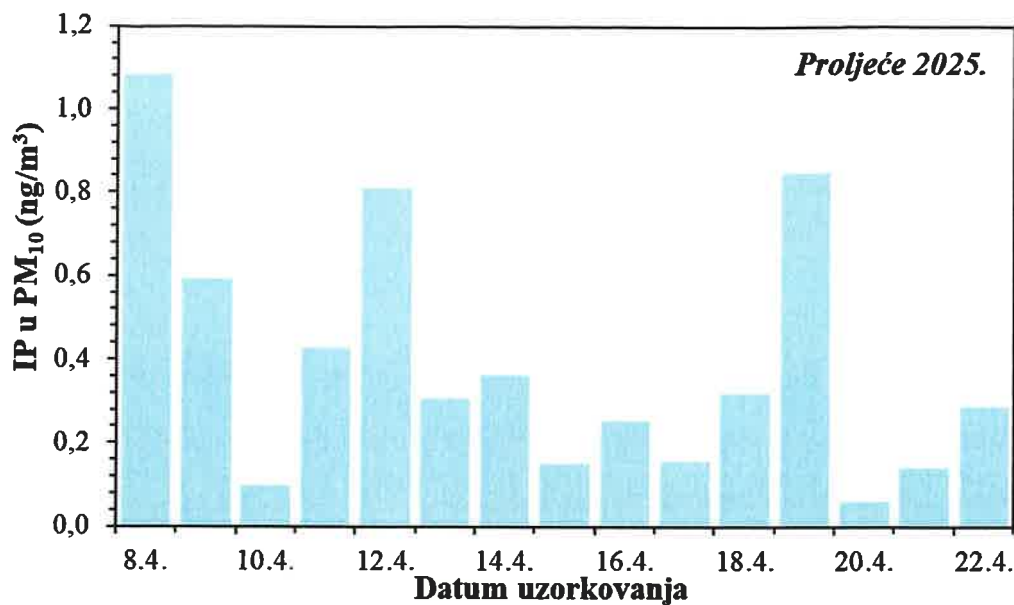
Slika 48. Kretanje srednjih dnevnih koncentracija IP u PM 10 frakciji lebdećih čestica na imisijskoj mjernoj postaji Jakuševac tijekom proljetnog razdoblja 2025. godine
