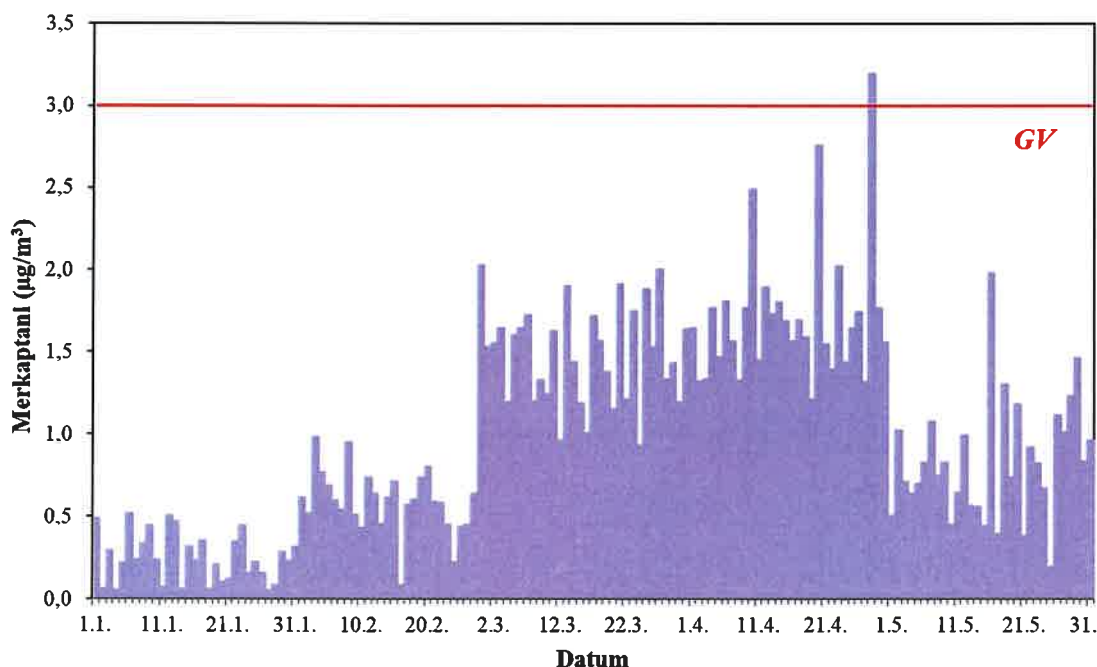
Slika 1. Kretanje srednjih dnevnih koncentracija merkaptana na mjernoj postaji u Jakuševcu od 1. siječnja do 31. svibnja 2025. godine
