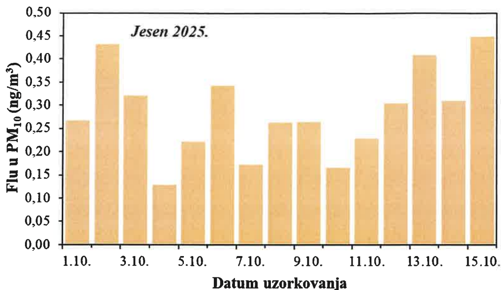
Slika 26. Kretanje srednjih dnevnih koncentracija Flu u PM 10 frakciji lebdećih čestica na imisijskoj mjernoj postaji Jakuševac tijekom jesenskog razdoblja 2025. godine
