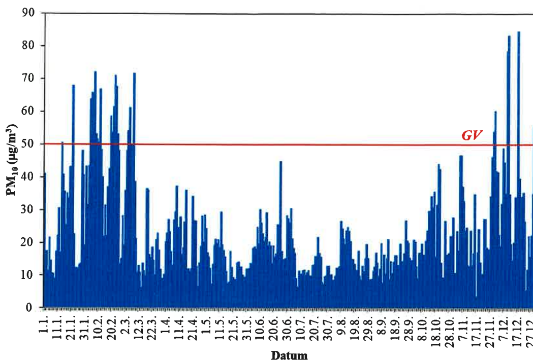
Slika 2. Kretanje srednjih 24-satnih koncentracija frakcije lebdećih čestica PM 10 tijekom 2025. godine
