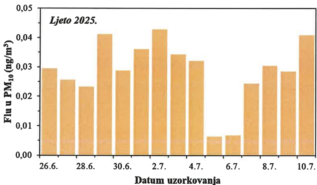
Slika 25. Kretanje srednjih dnevnih koncentracija Flu u PM 10 frakciji lebdećih čestica na imisijskoj mjernejoj postaji Jakuševac tijekom ljetnog razdoblja 2025. godine
