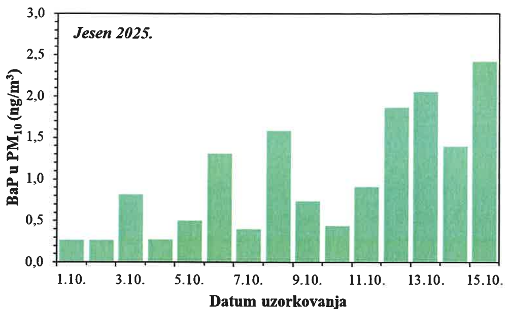
Slika 22. Kretanje srednjih dnevnih koncentracija BaP u PM 10 frakciji lebdećih čestica na imisijskoj mjernoj postaji Jakuševac tijekom jesenskog razdoblja 2025. godine
